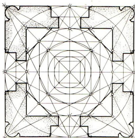
Ismoil Somoniy maqbarasining dynamik kvadratlar to'rida joylashgan tarhi.
