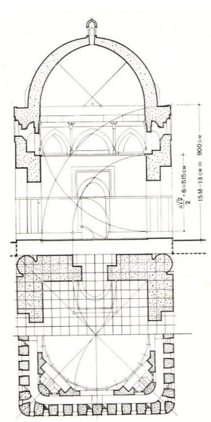
Ismoil Somoniy maqbarasi tarhi va qirqimi.
