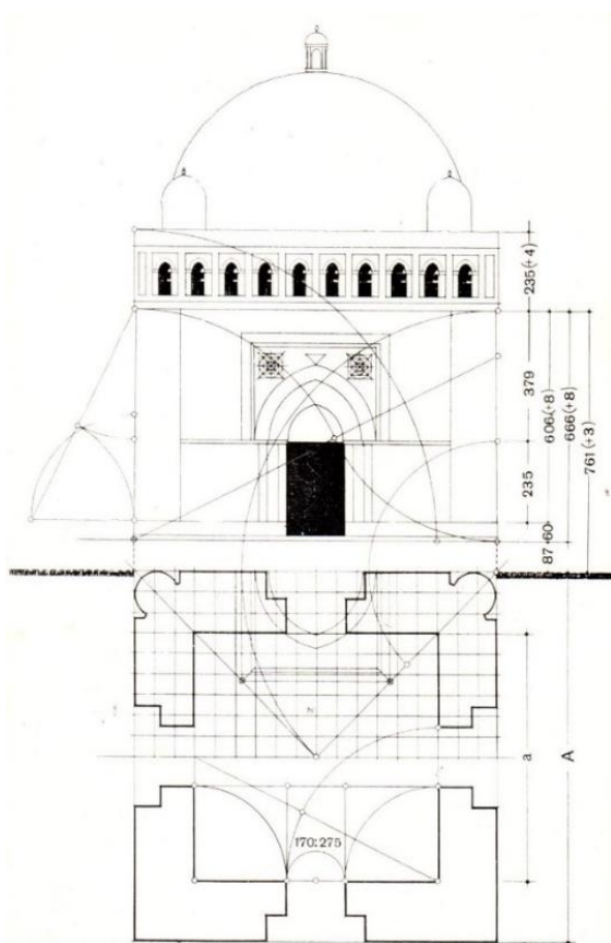
Ismoil Somoniy maqbarasi tarhi va qirqimi.
